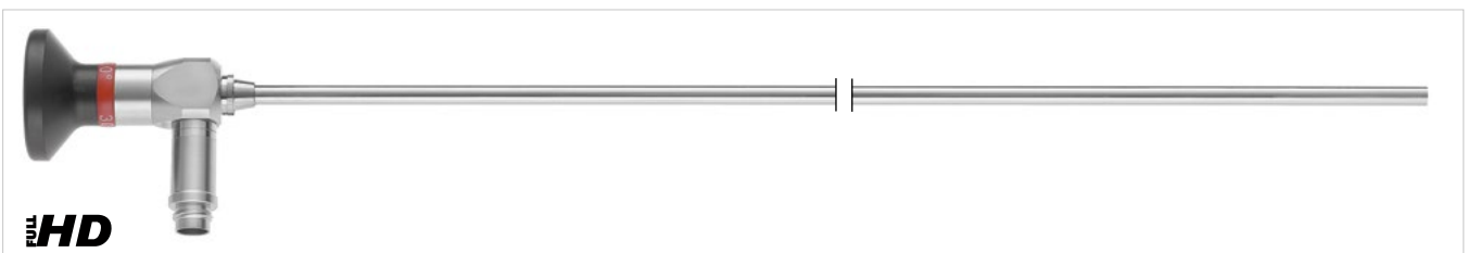
100-655-000 Nutzlänge 490 mm/working length 19 1/3 inch Bronchoskop, starr, 0°, ø 5,5 mm, autoklavierbar Bronchoscope, rigid, 0°, ø 5.5 mm, autoclavable
