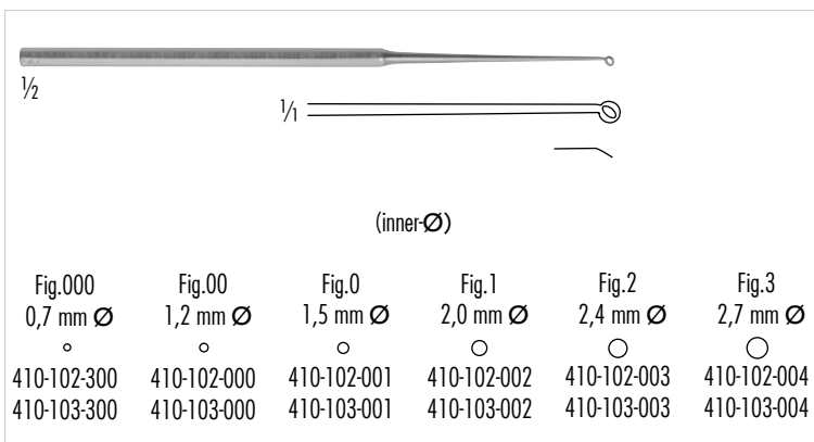
stumpf/blunt scharf/ sharp 410-102-000 410-103-000 410-102-001 410-103-001 410-102-002 410-103-002 410-102-003 410-103-003 410-102-004 410-103-004 410-102-300 410-103-300
