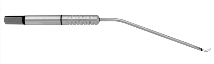
100-866-230 Tonsillennadel, bipolare Elektrode, stumpf, Nutzlänge 230 mm Tonsil bipolar electrode, blunt, working length 9 inch
