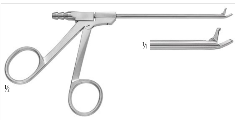
252-502-145 Biopsie Zange mit Absaugung, 2mm breit, durchschneidend, 45° aufwärts gebogen, Arbeitslänge: 100mm Biopsy Forceps with suction, 2mm wide, through-cutting, 45° upcurved, working length: 4 inch
